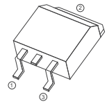
BT151K TO-263
